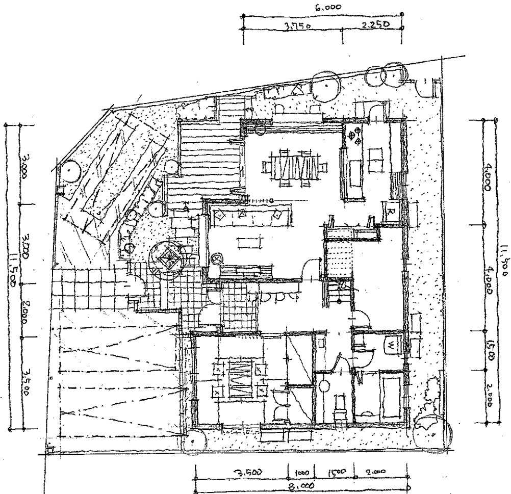
1層平面図 S: 1/100
