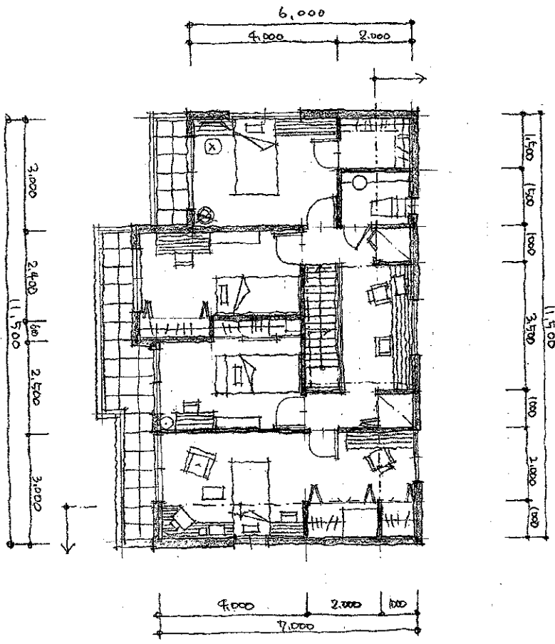
2層平面図 S: 1/100
